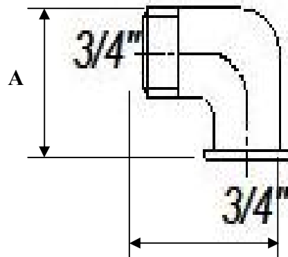
Фиг. 3. Коляно 90° М/Ж - 3/4"-3/4"
