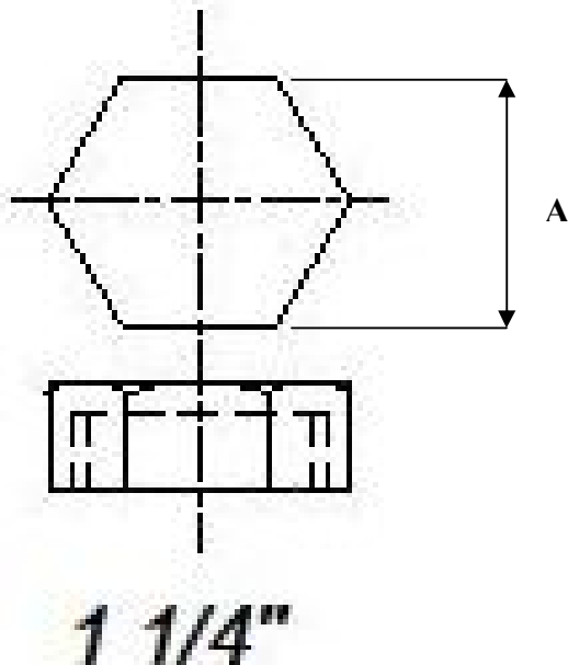
Фиг. 6. Капа Ж – 1 ¼" Размер А – от 40 мм до 50 мм
